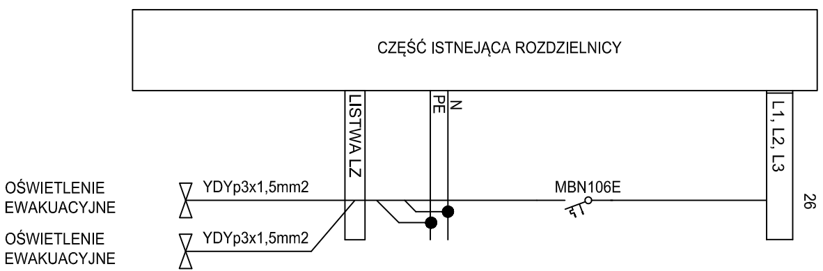
ROZDZIELNICA "R0"
