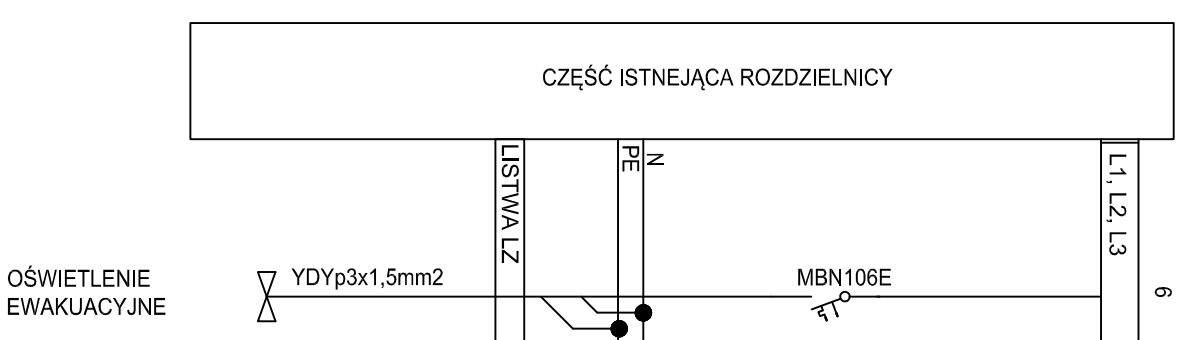
ROZDZIELNICA "R7"
