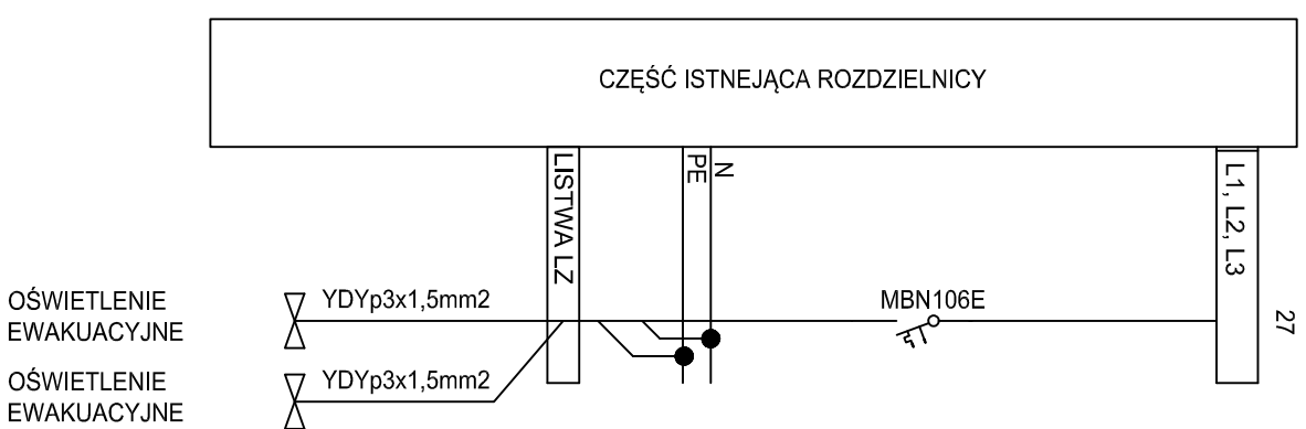
ROZDZIELNICA "R2"
