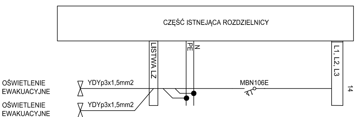
ROZDZIELNICA "R4"
