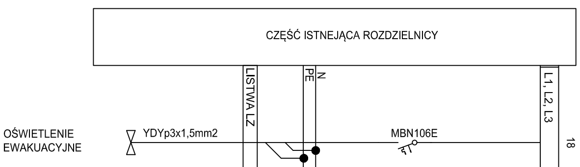
ROZDZIELNICA "R3"
